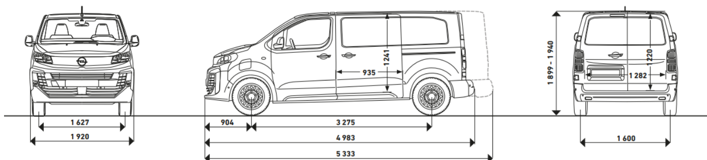
Rozměry VIVARO ELECTRIC VAN
